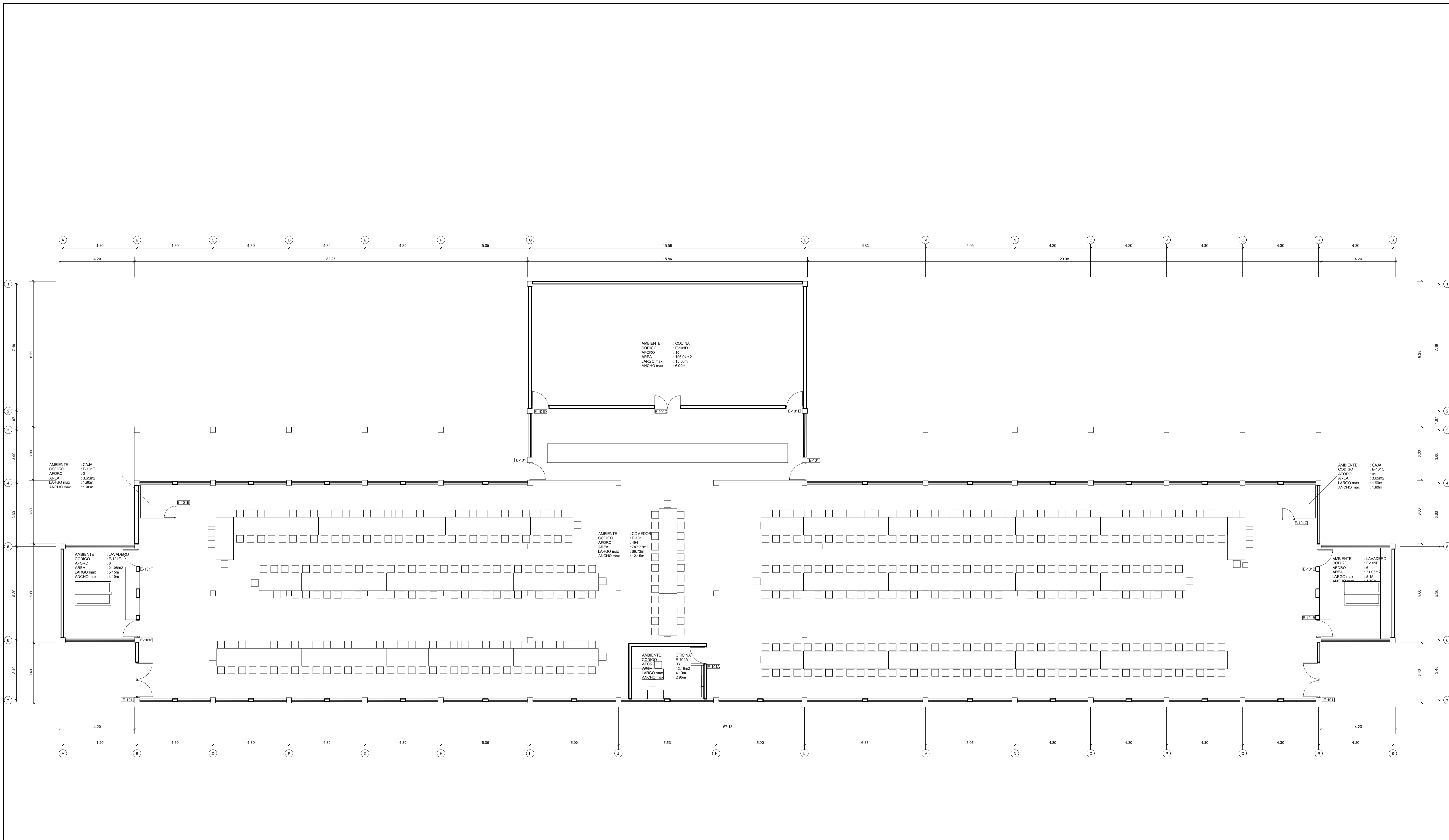
PRIMERA PLANTA AREA TECHADA = 1271.08m 2 AFORO = 524 ESCALA 1:100
